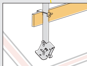
Applicazione su piano inclinato Application under the inclined floor
