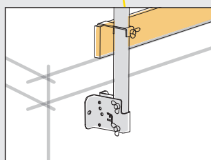
Applicazione a sbalzo Application on the surface
