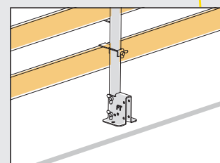
Applicazione staffa porta tavola Application bracket supporting
