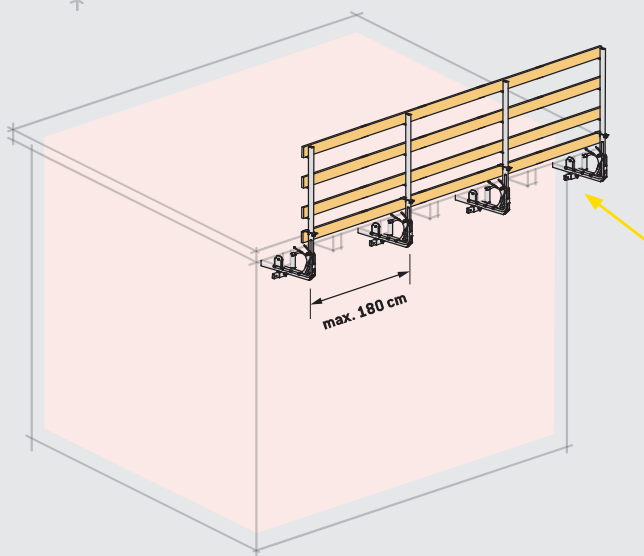
Applicazione su trave orizzontale. Application on horizontal beam.
