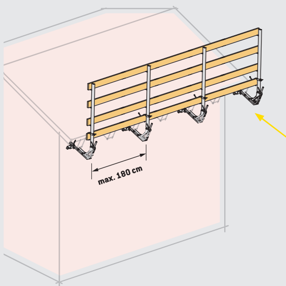
Applicazione su trave inclinata. Application on inclined beam.
