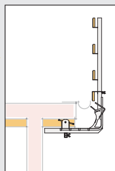
Applicazione su trave orizzontale. Application on horizontal beam.
