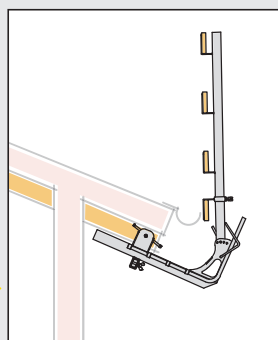
Applicazione su trave inclinata. Application on inclined beam.
